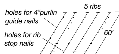
Fig. 5. Rib layout.
